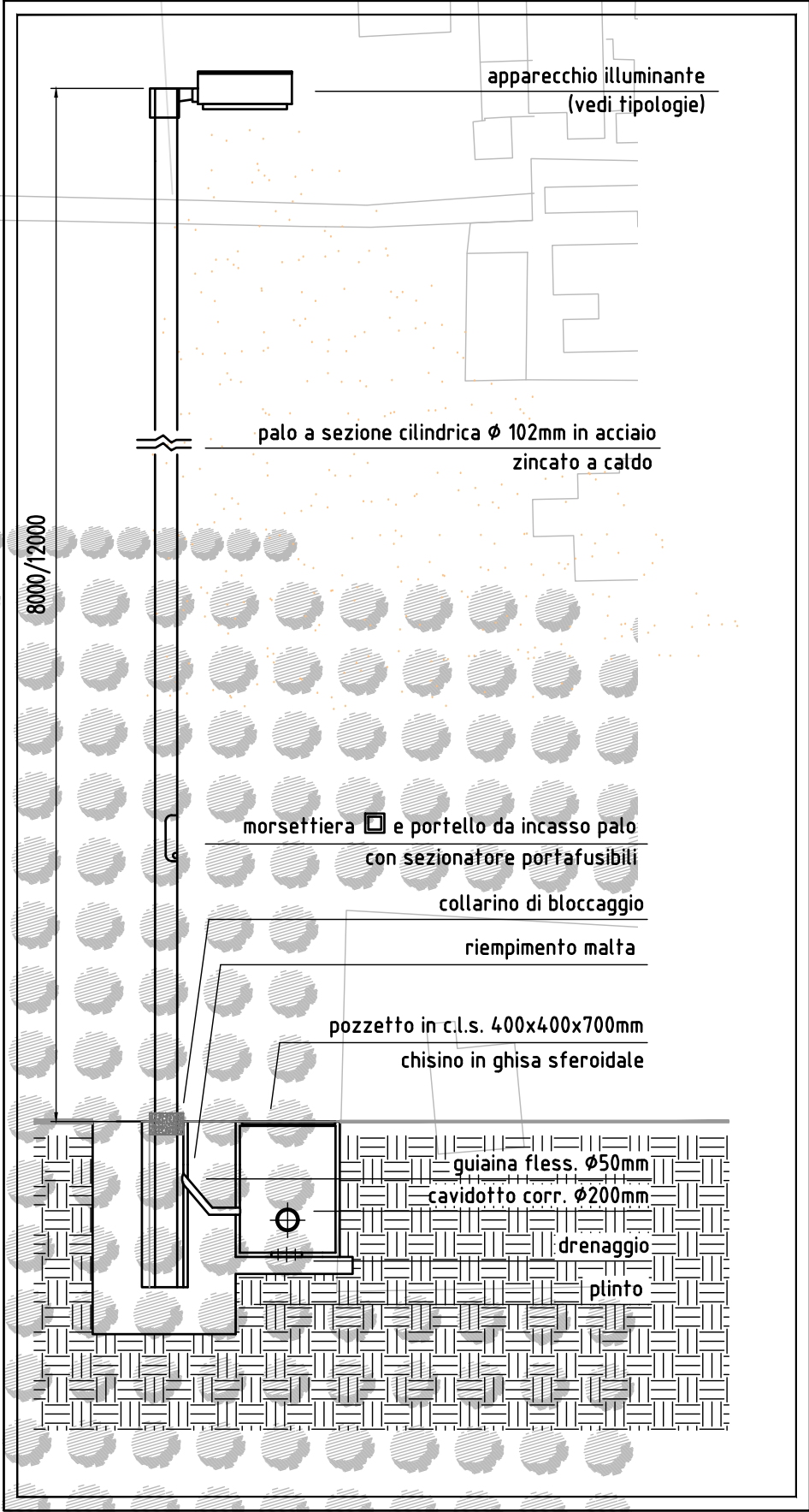
PARTICOLARE PREDISPOSIZIONE PER FUTURA INSTALLAZIONE PROIETTORE SU PALO
