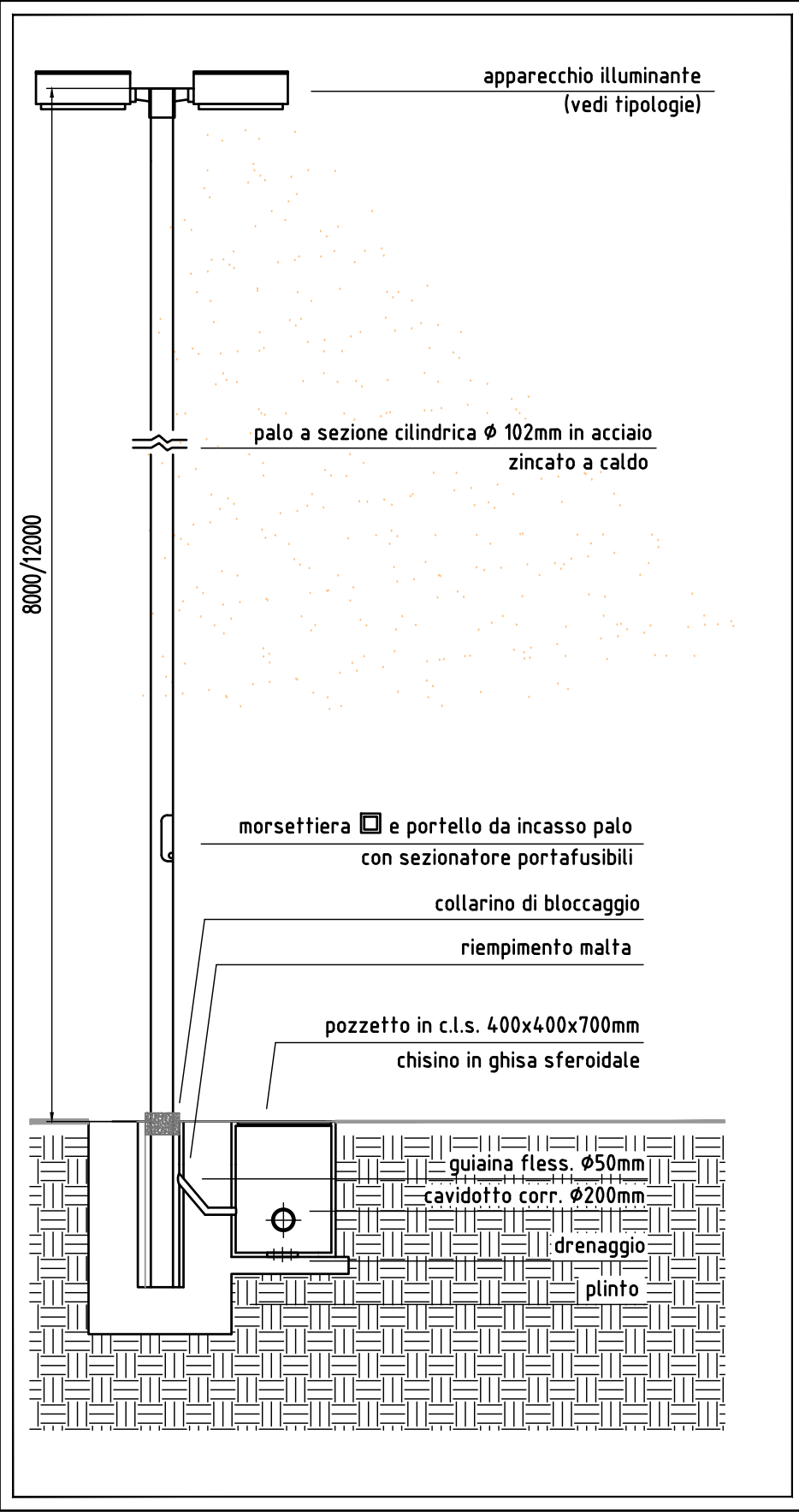
PARTICOLARE PREDISPOSIZIONE PER FUTURA INSTALLAZIONE DI N.2 PROIETTORI SU PALO
